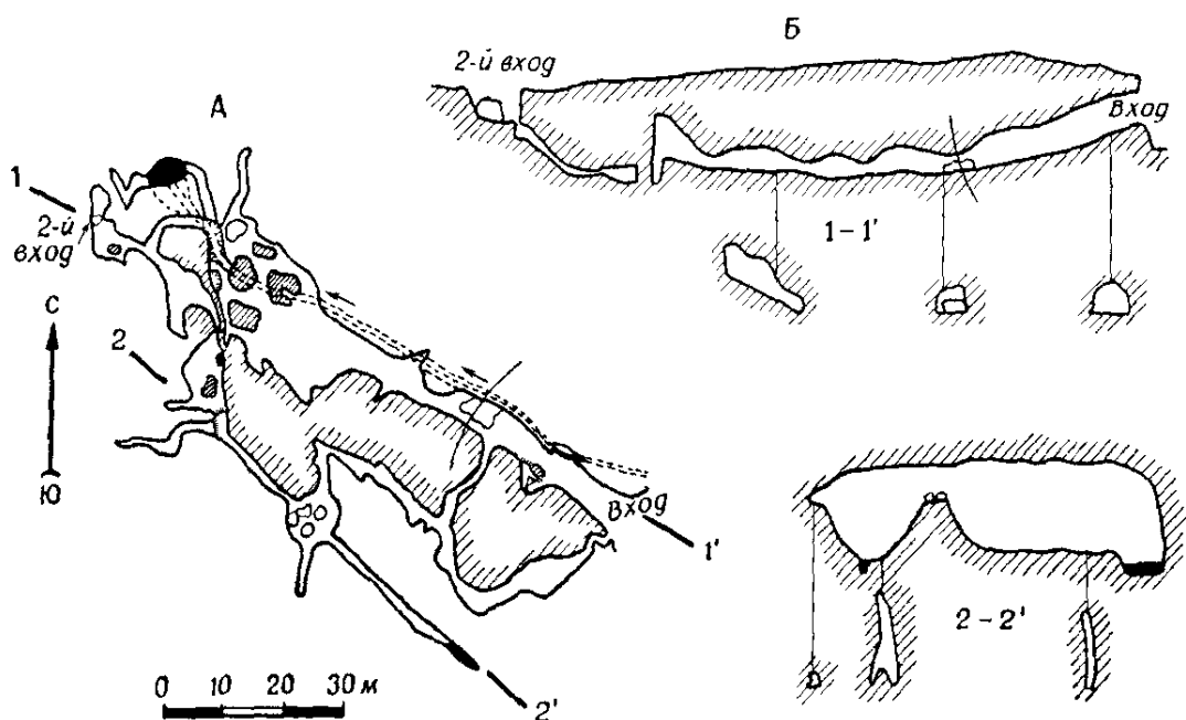
Рис. 10. Пещера Дружба. Съёмка СГС, 1963 г. Составили Э. Г. Лобанова и Б. Б. Поляков
