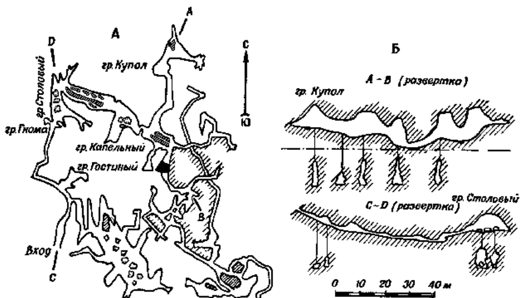
Рис. 20. Пещера Сказка. Съёмка СГС, 1967 г. Составили Н. Н. Сизова и В. О. Щелетов
