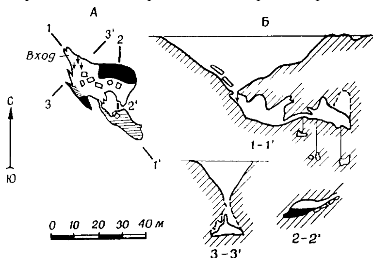
Рис. 8. Шахта Орловский провал. Съёмка СГС, 1962, 1965 гг. Составили В. О. Щепетов и Д. А. Круглов
