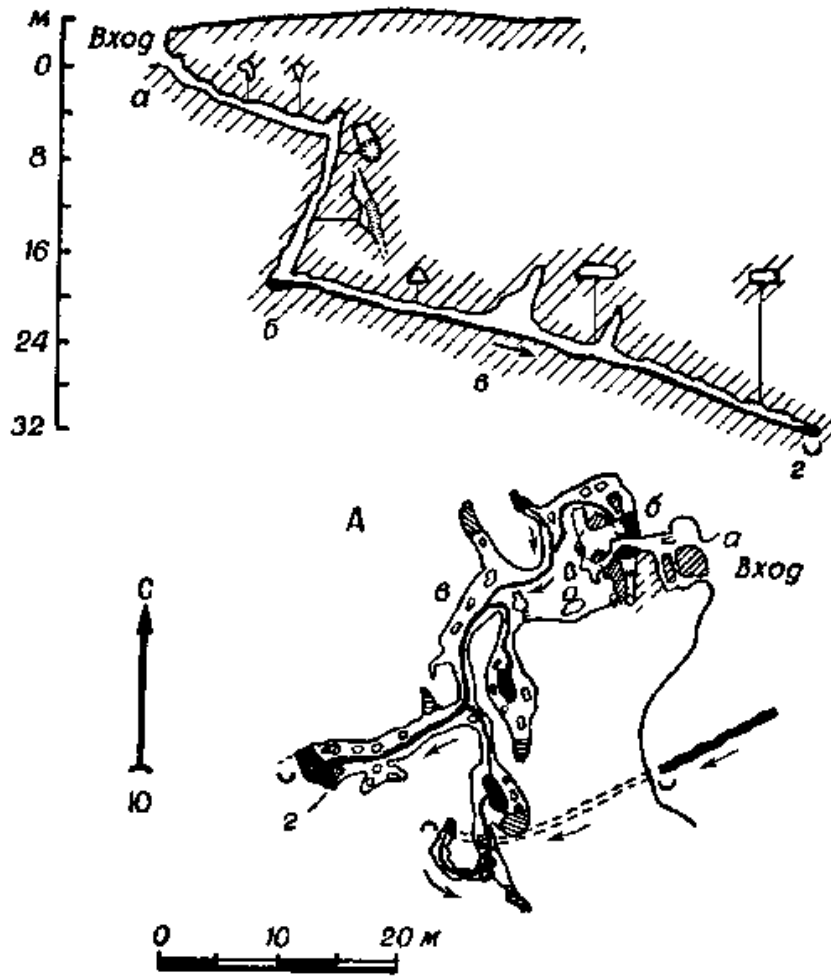
Рис. 16. Пещера Верхняя Провальная. Съёмка СГС, 1962, 1965 гг. Составили В. О. Щепетов и Г. Ф. Коваленко
