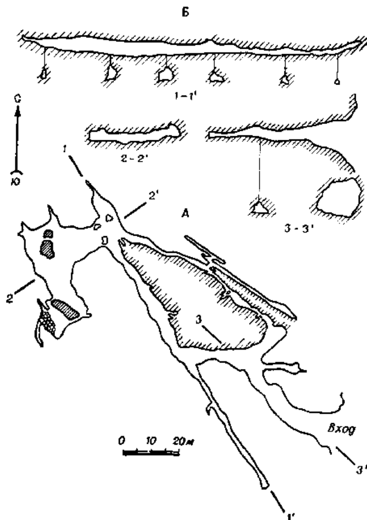
Рис. 5. Игнатовская пещера. Съёмка СГС, 1965 г. Составил Г. Ф. Коваленко
