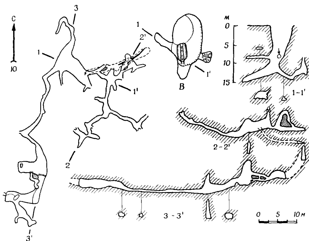
Рис. 13. Пещера Глиняная. Съёмка СГС, 1962 г. Составил В. О. Щепетов
