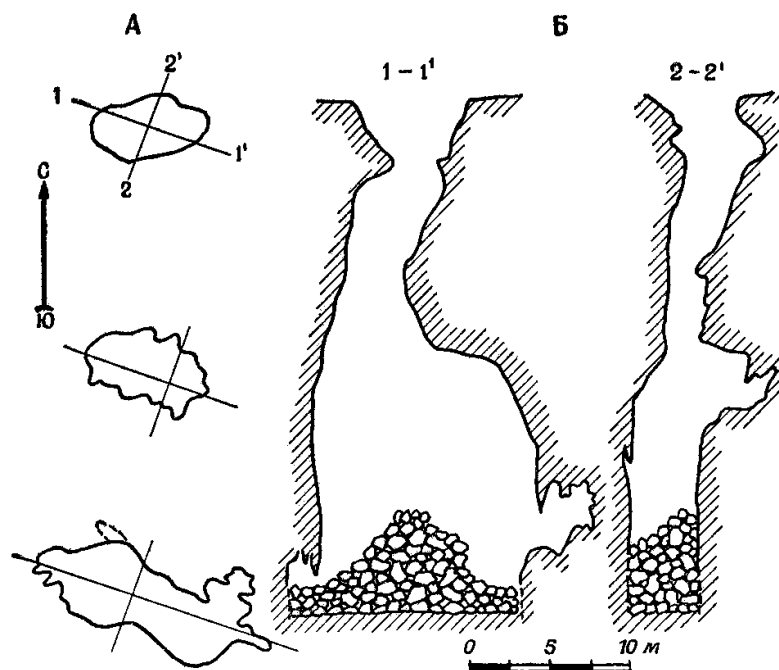
Рис. 21. Шахта Иргизлинская. Съёмка СГС, 1967. Составила Н. Н. Сизова
