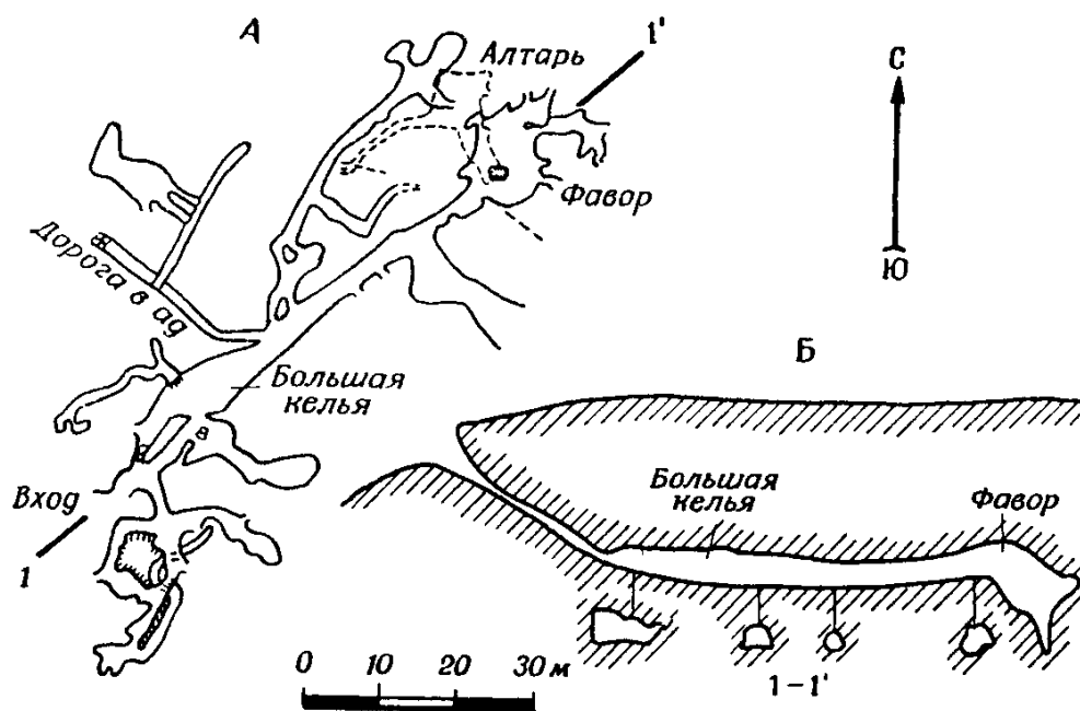
Рис. 26. Пещера Смолинская. Съемка СГС, 1962 г. Составили Б. Б. Поляков и В. О. Щепетов
