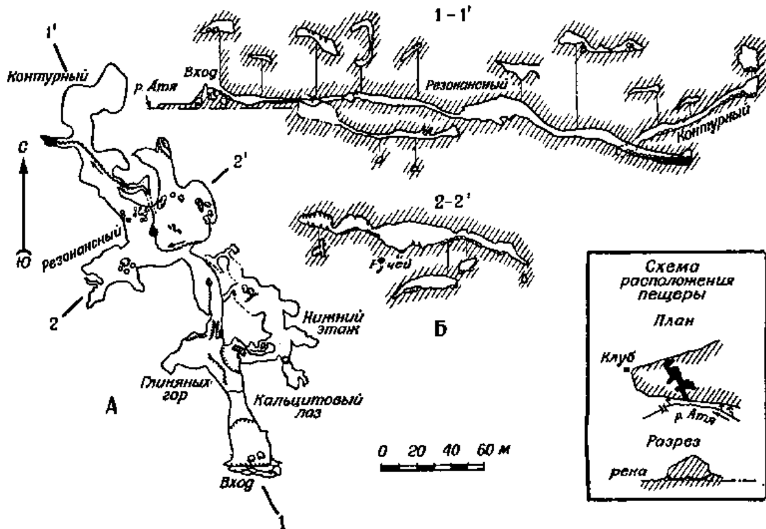
Рис. 6. Пещера Сухая Атя. Съемка СГС, 1963 г. Составили А. Ф. Рыжков, Б. Б. Поляков.
