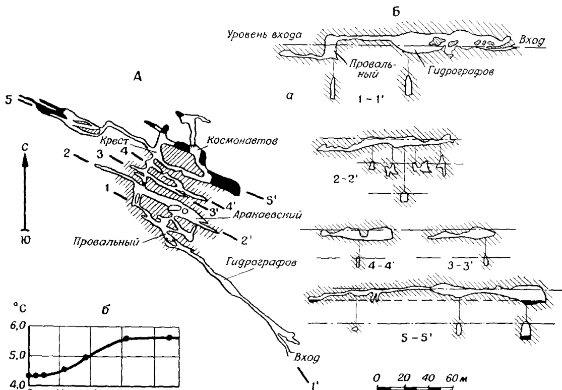
Рис. 23. Пещера Максимовича. Съёмка СГС, 1963 г. Составили Э. Г. Лобанова и Л. Ф. Емельянов
