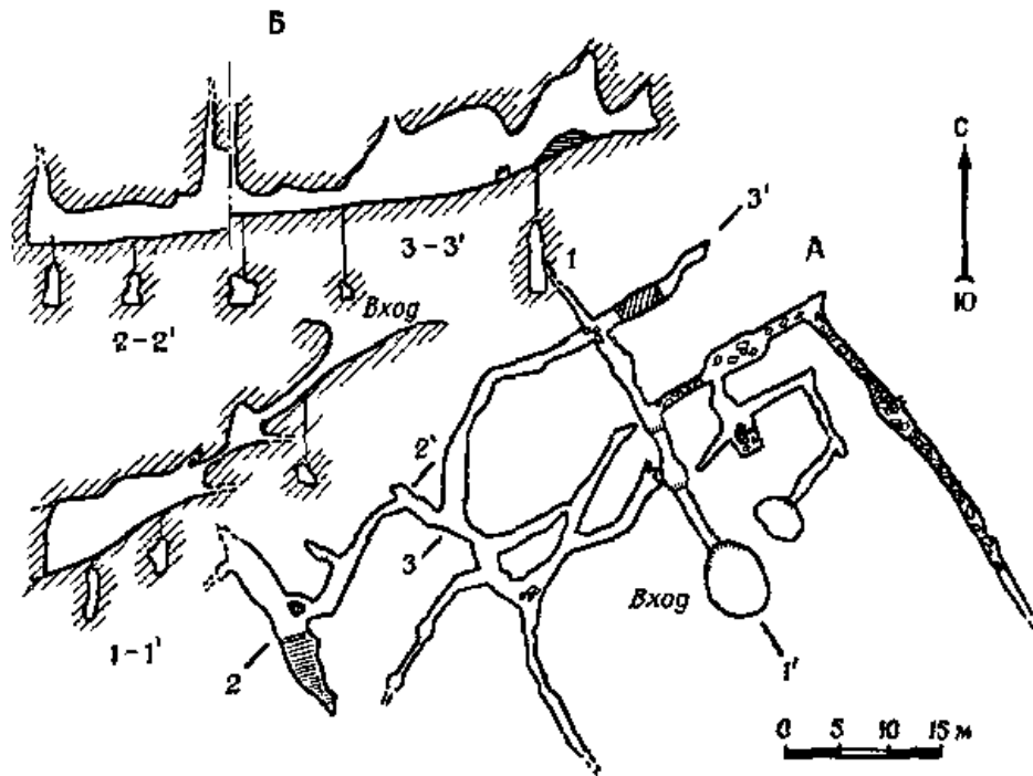
Рис. 15. Минская пещера. Съёмка СГС, 1963, 1965 гг. Составили В. О. Щепетов и А. Г. Седышев
