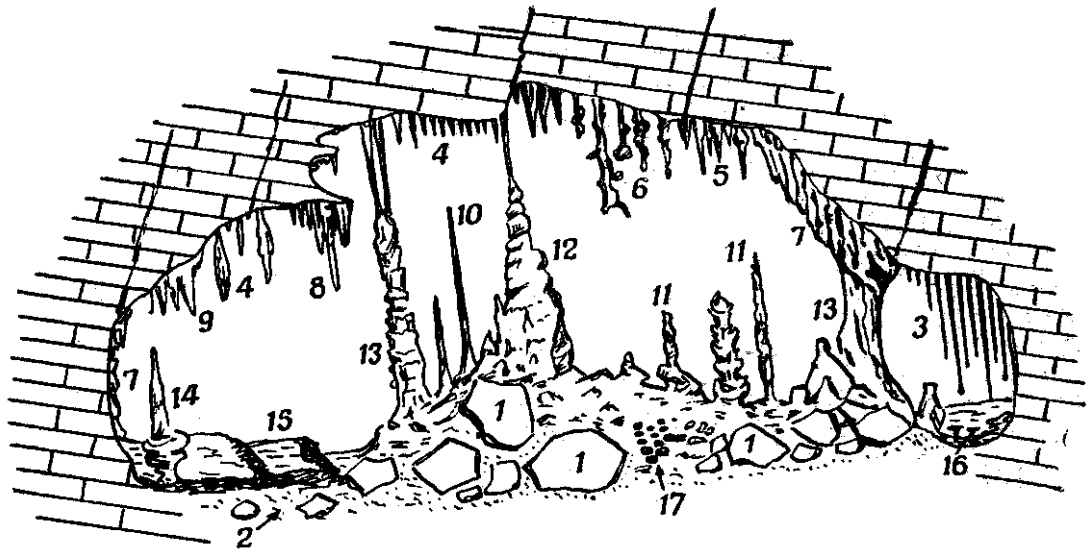
Рис. 1. Обобщенная схема пещерных отложений (составила К. А. Горбунова):
