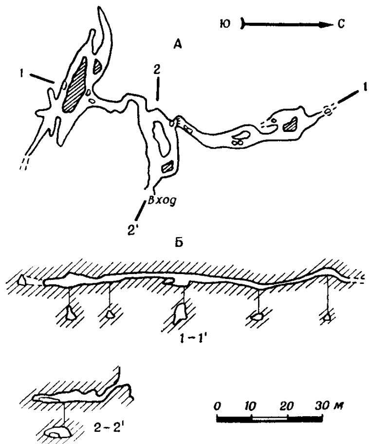
Рис. 9. Катниковская пещера. Съёмка СГС, 1962 г. Составили Э. Г. Лобанова и Л. Ф. Емельянов
