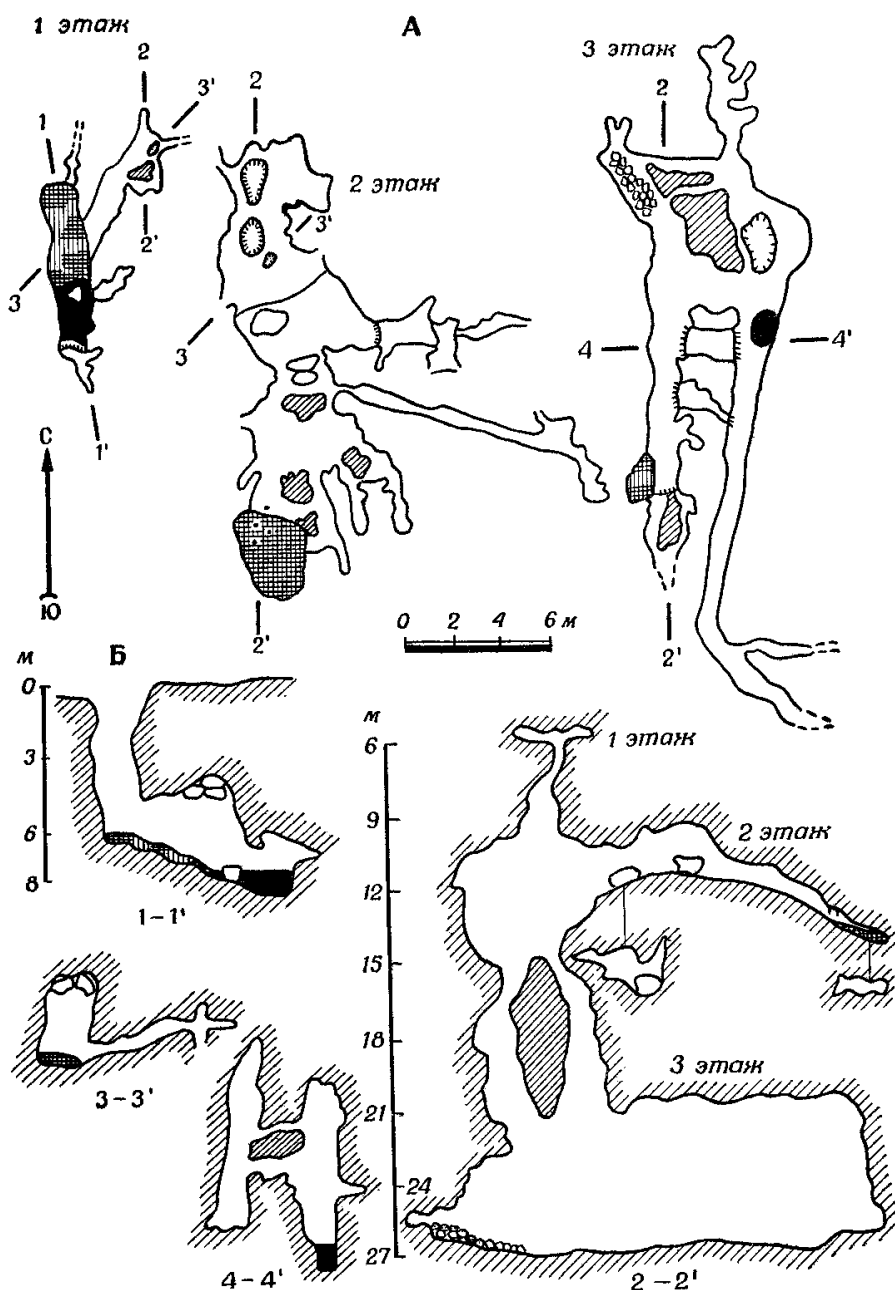
Рис. 25. Шахта Светлая. Съёмка СГС, 1964 г. Составили В. И. Кузнецов и А. Г. Седышев
