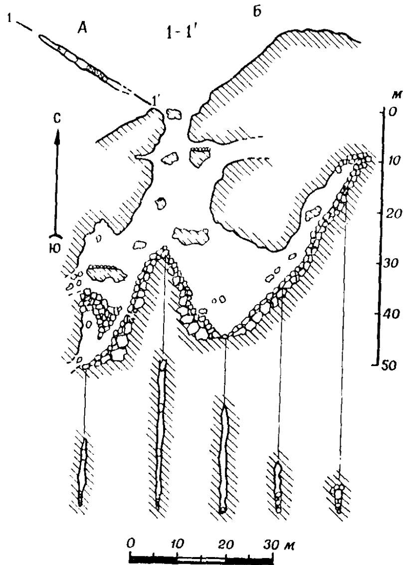
Рис. 3. Шахта Саранская. Съемка Свердловской городской спелеосекции (СГС), 1965 г. Составили В. И. Кузнецов и А. Г. Седышев. Здесь и далее на планах меридиан магнитный. Условные обозначения по Максимовичу — Дублянскому. А — план, Б — профиль
