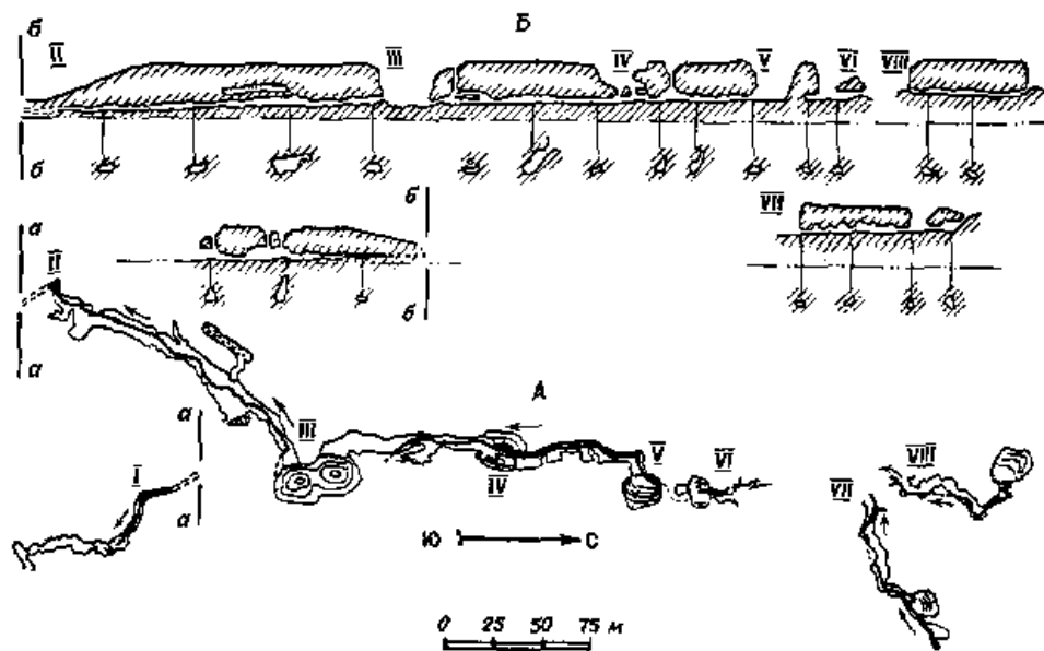
Рис. 7. Ижемская пещерная система. Съёмка СГС, 1964 г. Составили Г. В. Васильев и В. И. Кузнецов
