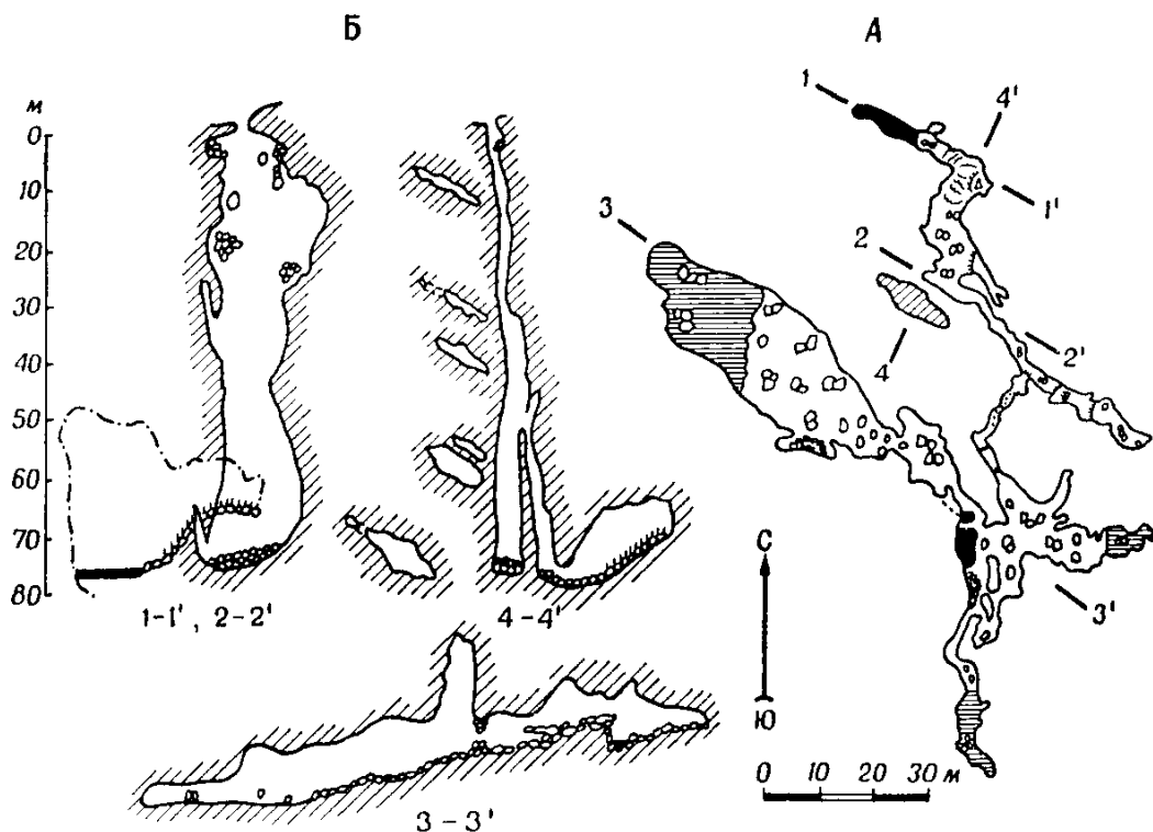
Рис. 18. Шахта Пропащая Яма. Съёмка СГС, 1967 г. Составили В. Д. Марков, Ю. Н. Логинов, А. М. Кабалин
