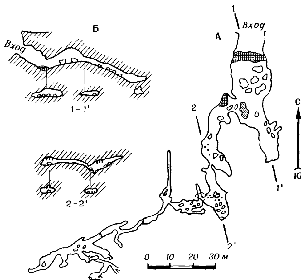
Рис. 11. Аракаевская пещера. Съемка СГС, 1962, 1965 гг. Составили В. О. Щепетов и В. И. Шагалов
